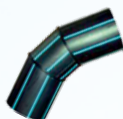
CURVA 45° SETTORE PE100 (MRS10) DERATING FACTOR 0,8 (COEFFICIENTE DI RIDUZIONE) NORME: EN 12201-3 racordi per distribuzione dell'acqua
