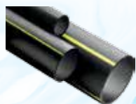
TUBO POLIETILENE PE100 ALTA DENSITÀ PER GAS COMBUSTIBILI NORMA UNI 1555
